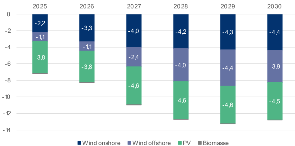
Abbildung 10: Geringere Investitionen bei Wind, Photovoltaik und Biomasse 2025-2030 (Mrd. Euro) bei um 25% verringertem Ausbauszenario
