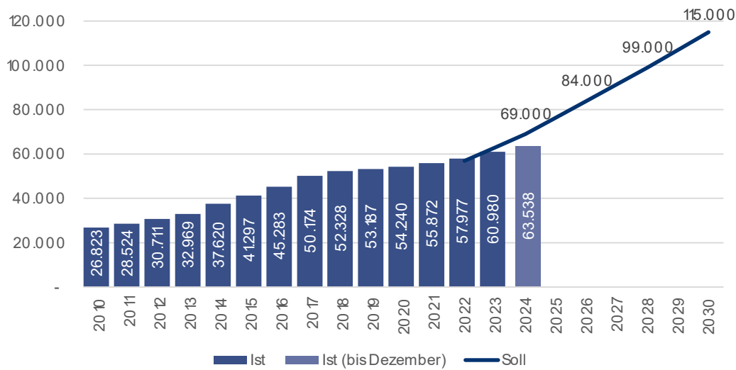
Abbildung 1: Ausbau der installierten Leistung von Windenergieanlagen (Onshore) in MW
