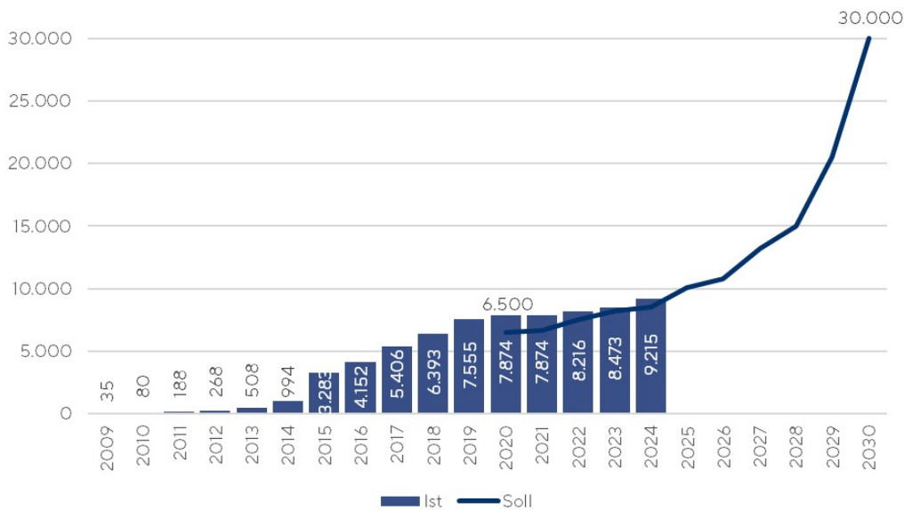
Abbildung 2: Ausbau der installierten Leistung von Windenergieanlagen (Offshore) in MW
